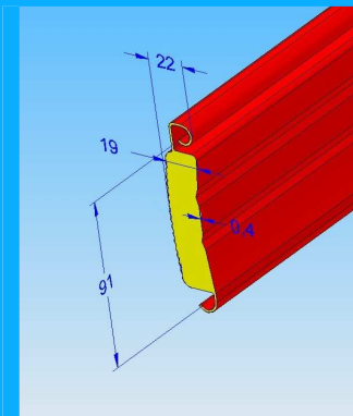
Τομή μονωτικού προφίλ
